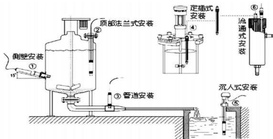
电极安装示意图
