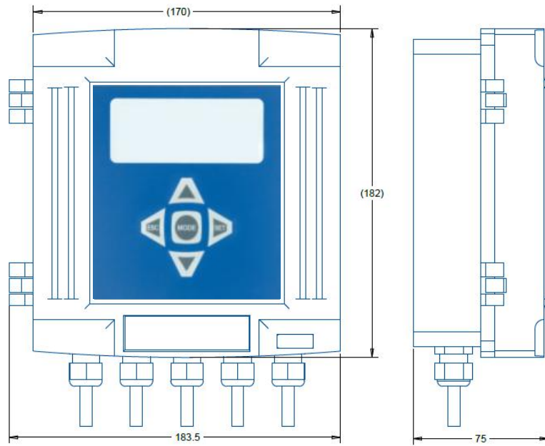
图 2-8 变送器尺寸图
