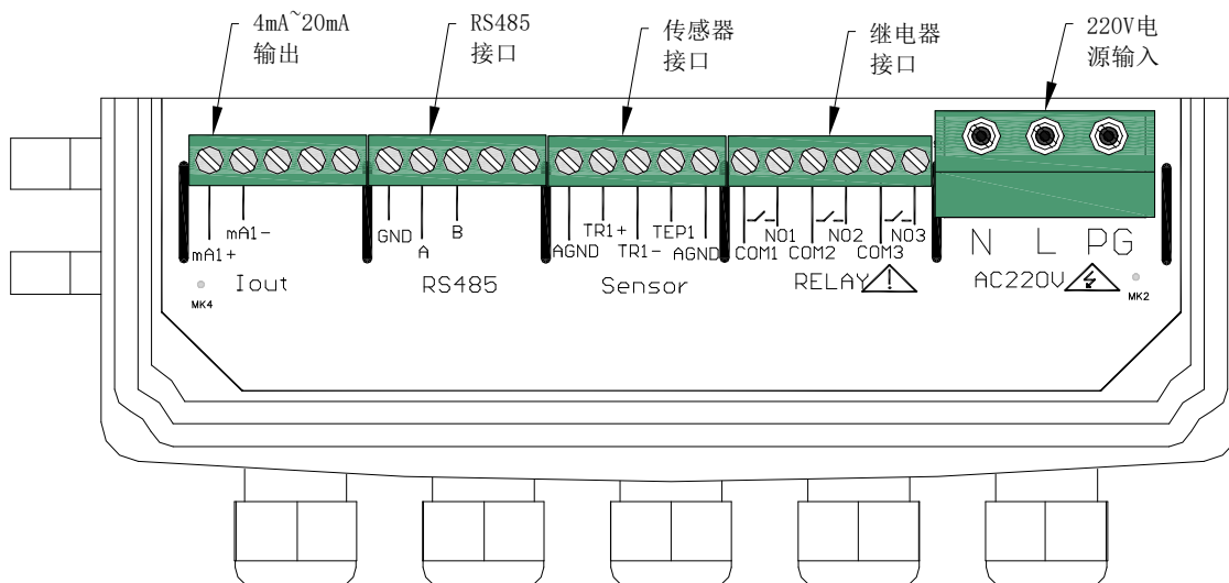
图 2-10 接线盒内部接线端子
