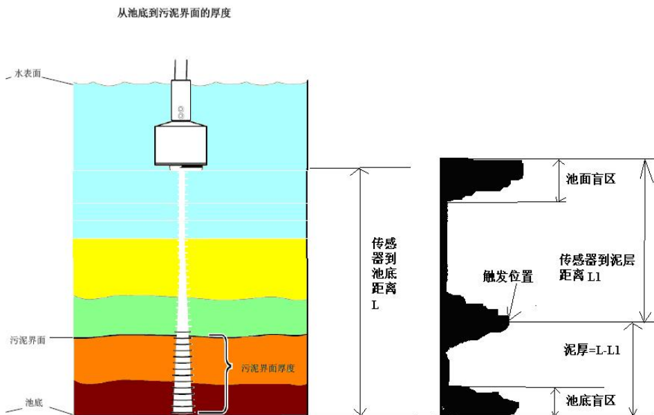
图 1-1 仪表工作原理
